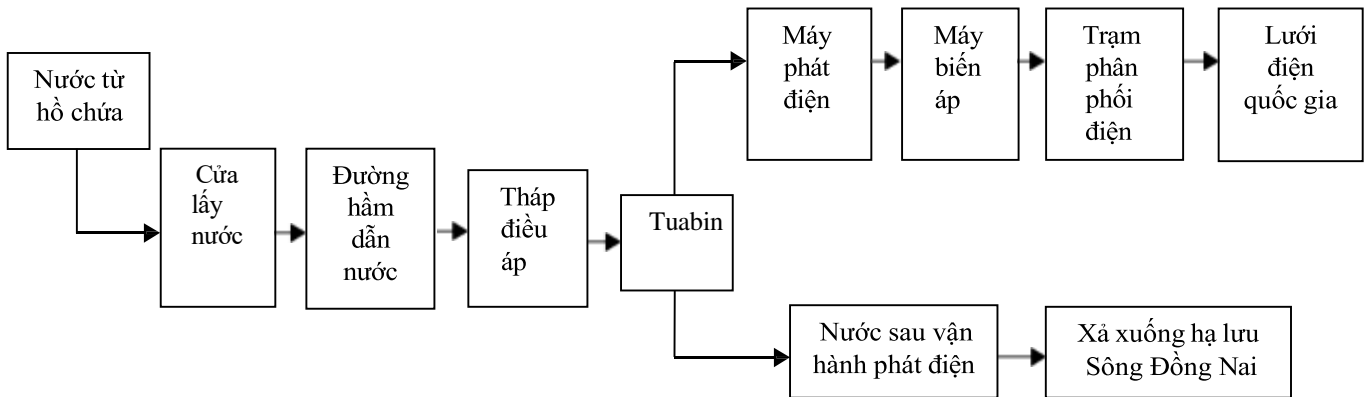
Hình 2. Sơ đồ quy trình sản xuất điện năng
